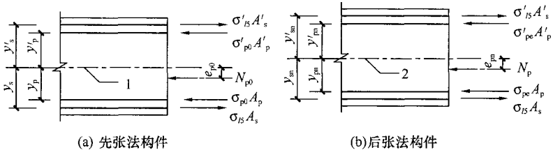
图 10.1.7 预加力作用点位置
