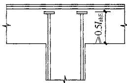
(f) 顶层中间节点柱筋加锚头(锚板)锚固
